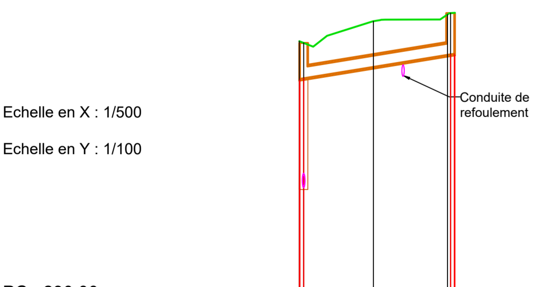
Rue de Lorraine : antenne DO 15
