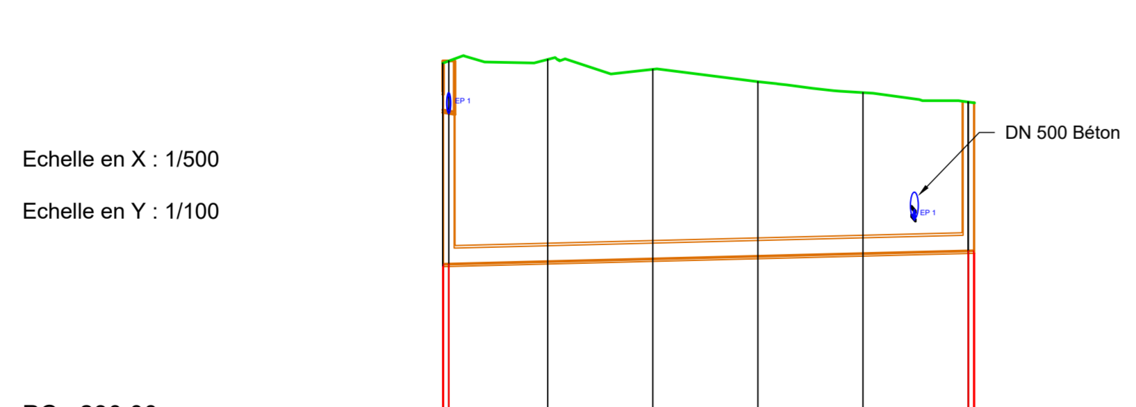
Rue de Lorraine : antenne DO 14
